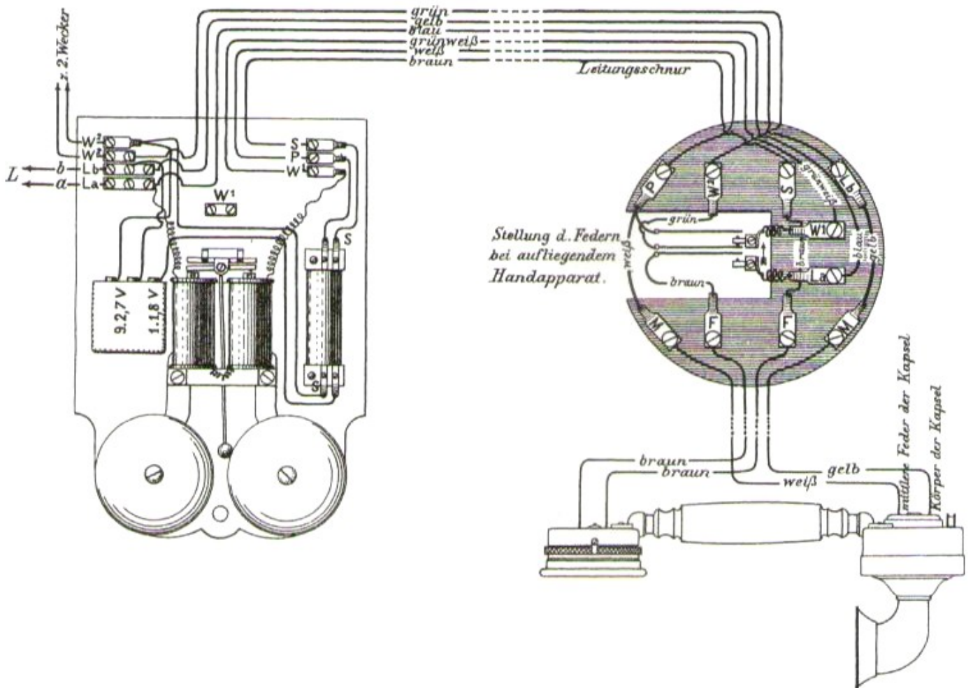
Fig. 29. Stromlauf.
