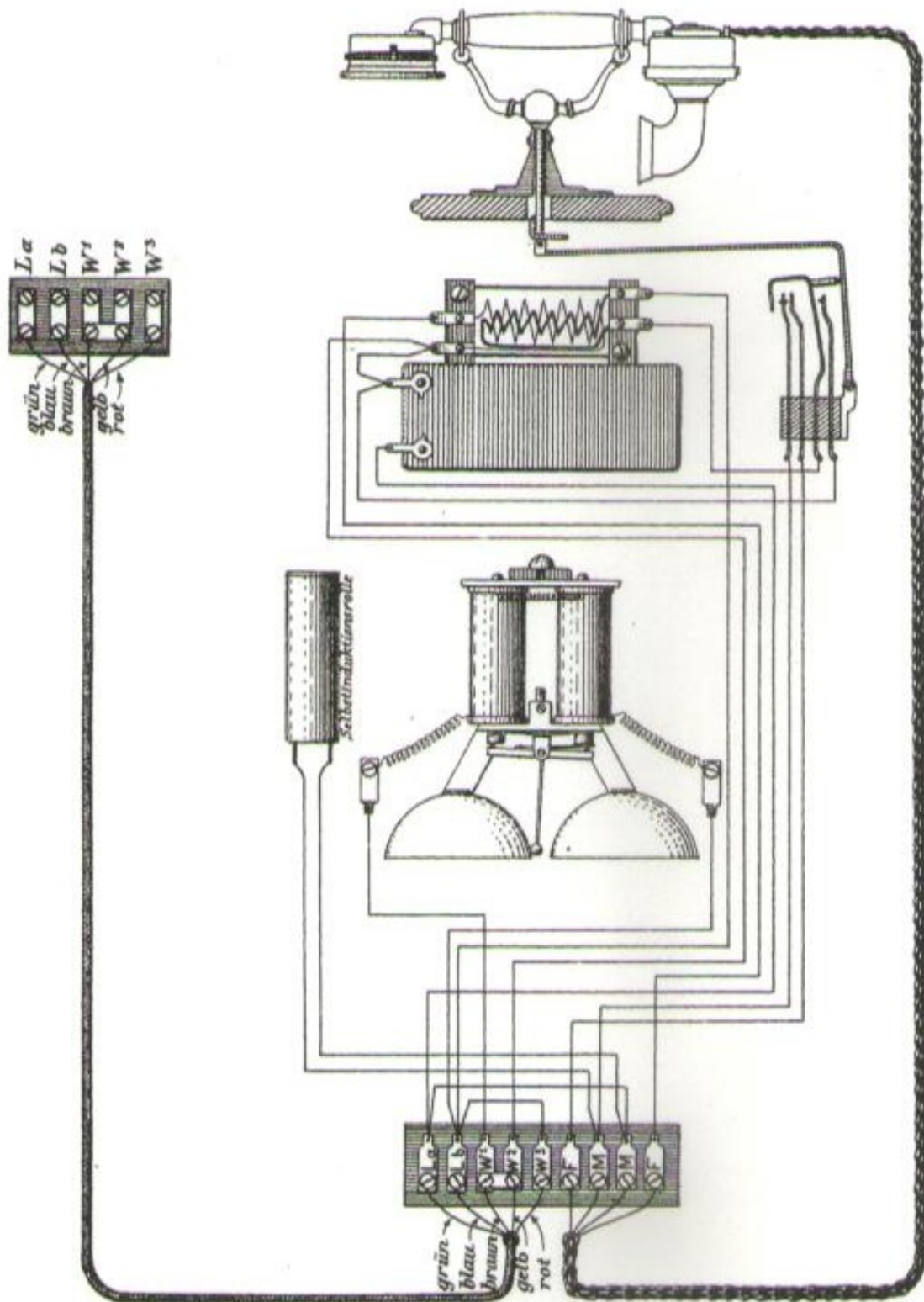
Fig. 30. Stromlauf.
